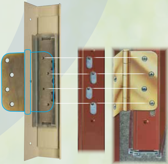
Inside Door Slab
